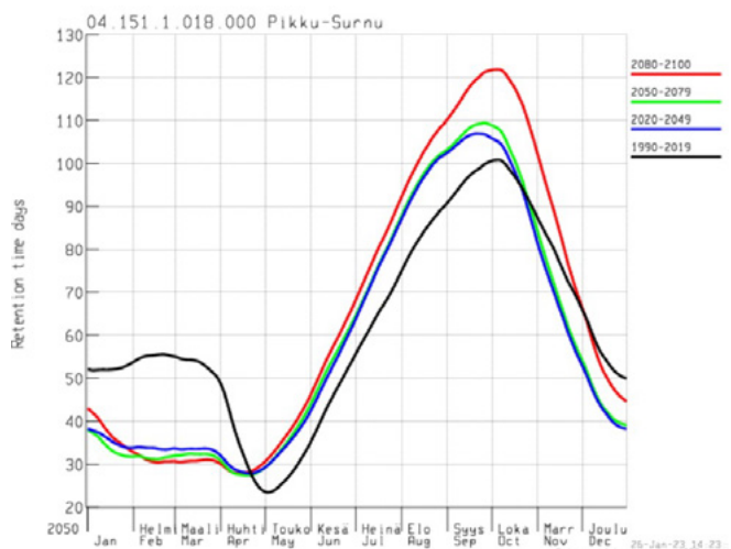
Kuva 7. Pikku-Surnun veden viipymä ilmastomalleilla SMHI RCA4 ja MPI-M-MPI-ESM-LR ja päästöskenaariolla RCP2,5 ennustettuna (SYKE WSFS-DEMALA, 2023).
