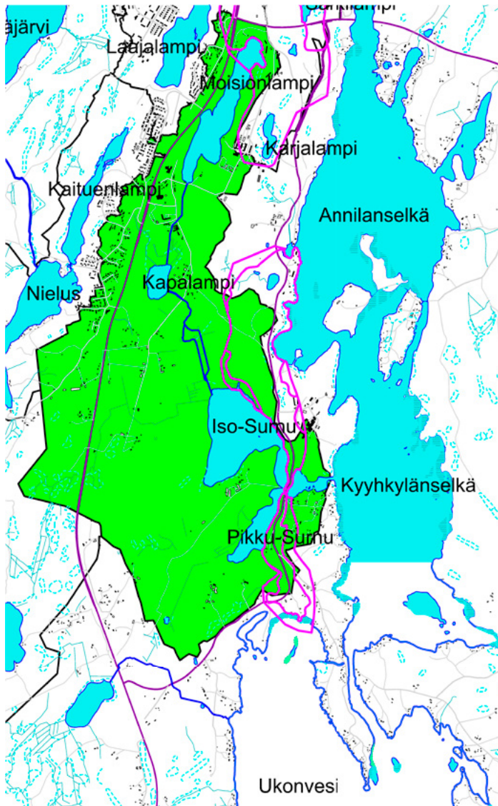
Kuva 3. Pikku-Surnun valuma-alue vihreällä. Porrassalmen pohjavesi-alueen rajaus violetilla. Valuma-alueeseen on nyt otettu mukaan myös Pikku-Surnun ja Kyyhkölän välinen salmi, jonka vesi voi päätyä takaisinvirtauksen vuoksi Pikku-Surnuun. On myös mahdollista, että salmesta tapahtuu rantaimetyymistä.
