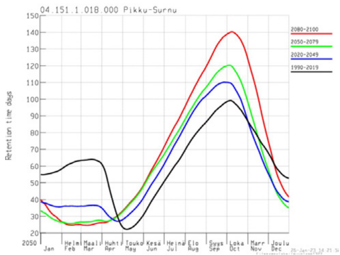
Kuva 6. Pikku-Surnun veden viipymä ilmastomalleilla SMHI RCA4 ja MOHC-HadGEM2-ES ja päästöskenaariolla RCP8,5 ennustettuna (SYKE WSFS-DEMALA, 2023).
