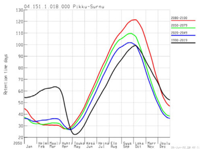
Kuva 8. Pikku-Surnun veden viipymä ilmastomalleilla SMHI RCA4 ja MPI-M-MPI-ESM-LR ja päästöskenaariolla RCP4,5 ennustettuna (SYKE WSFS-DEMALA, 2023).
