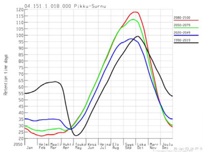
Kuva 9. Pikku-Surnun veden viipymä ilmastomalleilla SMHI RCA4 ja MPI-M-MPI-ESM-LR ja päästöskenaariolla RCP8,5 ennustettuna (SYKE WSFS-DEMALA, 2023).
