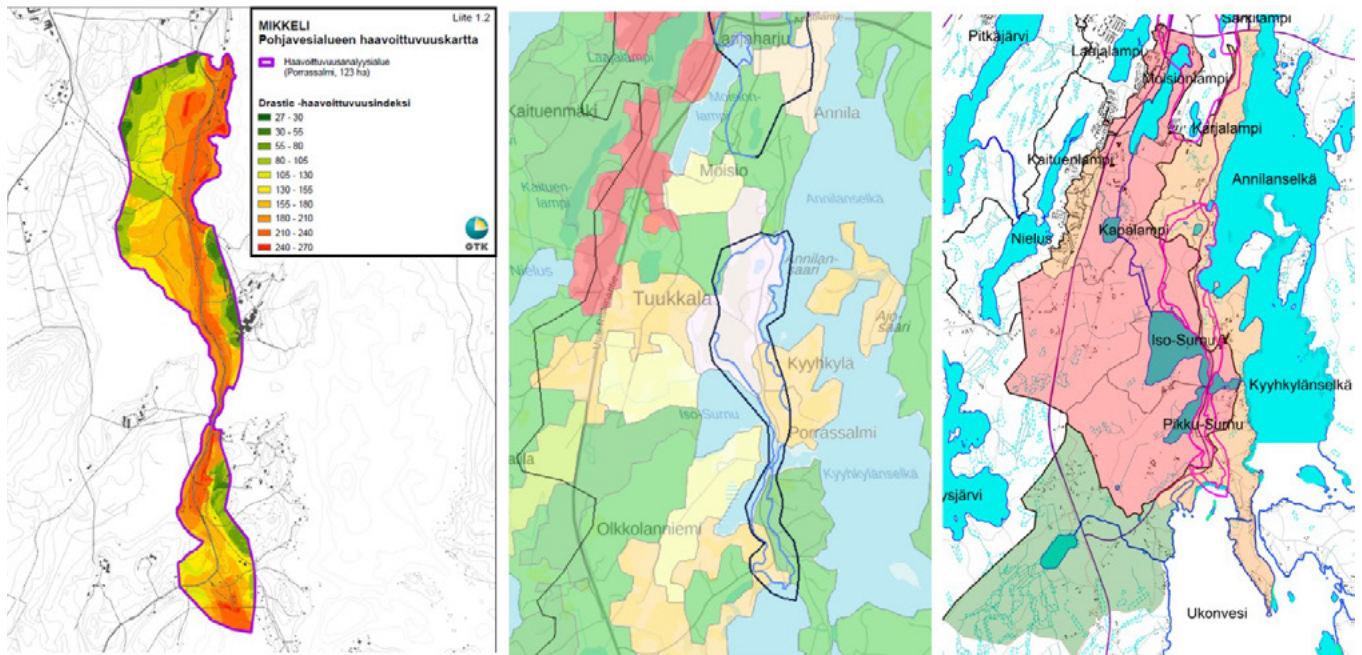
Kuva 52. Keskellä Corine maankäyttöluokat, jossa vihreät alueet ovat metsää. Vasemmalla DRASTIC-haavoittuvuusanalyysi ja oikealla rantaimetyymisaluiden haavoittuvuusanalyysi. (Hyvönen & Luoma, 2019; Maanmittauslaitos, paikkatietoikkuna, 2023.)
